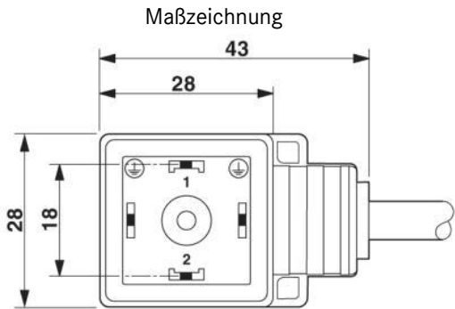
Ventilstecker, Bauform A
