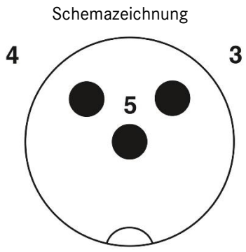
Polbild M12-Stecker, 3-polig, A-kodiert, Ansicht Stiftseite
