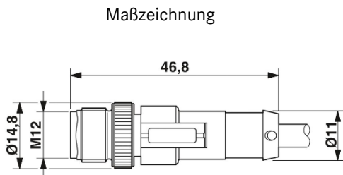
Stecker M12 x 1, gerade, geschirmt, A-kodiert
