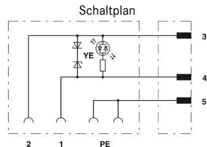
Kontaktbelegung des M12-Steckers und des Ventilsteckers
